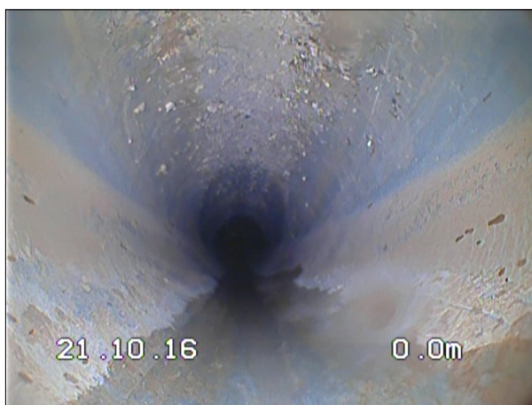
Photo: 9_9_9_A.jpg, 00:00:01 0m, Noeud de départ, regard de visite Eu 1
