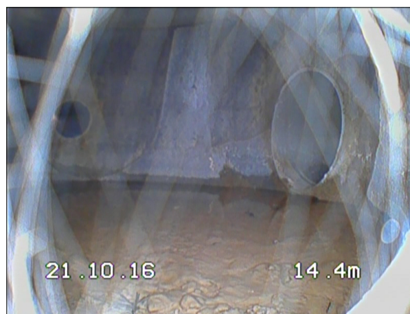
Photo: 2_2_14_A.jpg, 00:00:24 14,4m, Noeud d'arrivée, regard de visite Ep 5
